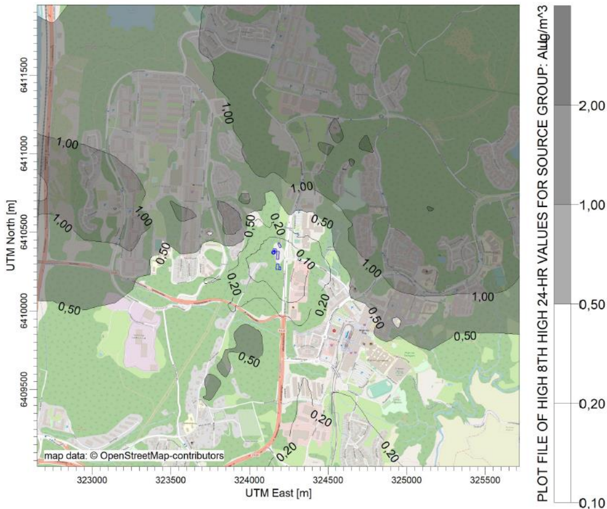
Figur 24: Haltbidrag av NO2 (dygnmedell) från ny anläggning med 100 m skorsten. Haltbidraget inkluderar både existerande skorstenar och ny skorsten.
