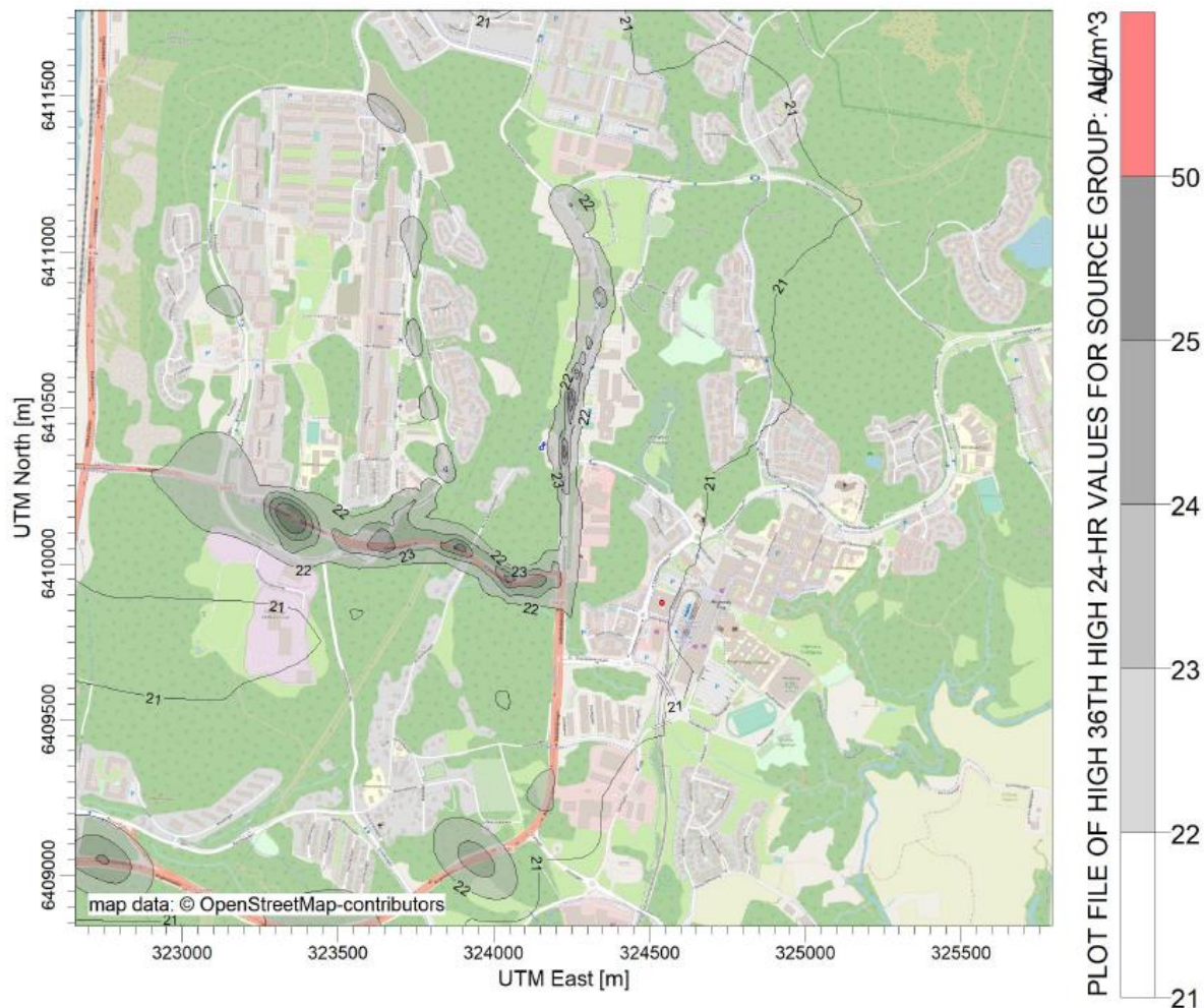
Figur 26: Dygnmedelvärde av totalhalt för partiklar för nollalternativet. MKN överskrids ej.
