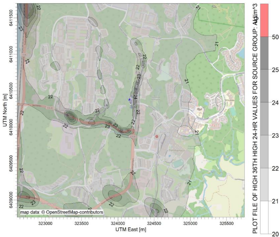
Figur 30: Dagnmedelvärde av totalhalt för partiklar för utredningsalternativet vid 70 m hög skorsten. MKN överskrids ej.
