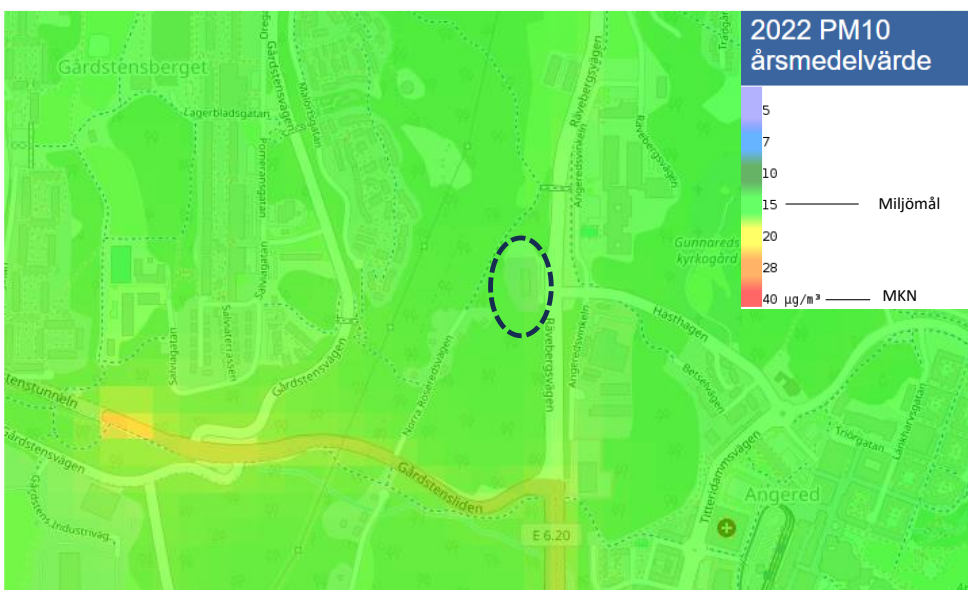
Figur 5. Årsmedelvärde av PM 10 vid värmeverket i Angered (Göteborgs Stad, 2024). Placering av värmeverket vid svart ring.
