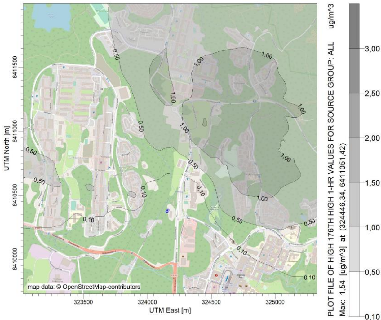
Figur 13: Haltbidrag av NO 2 (timmesmedel) för existerande anläggning, utan trafik och bakgrundshalter
