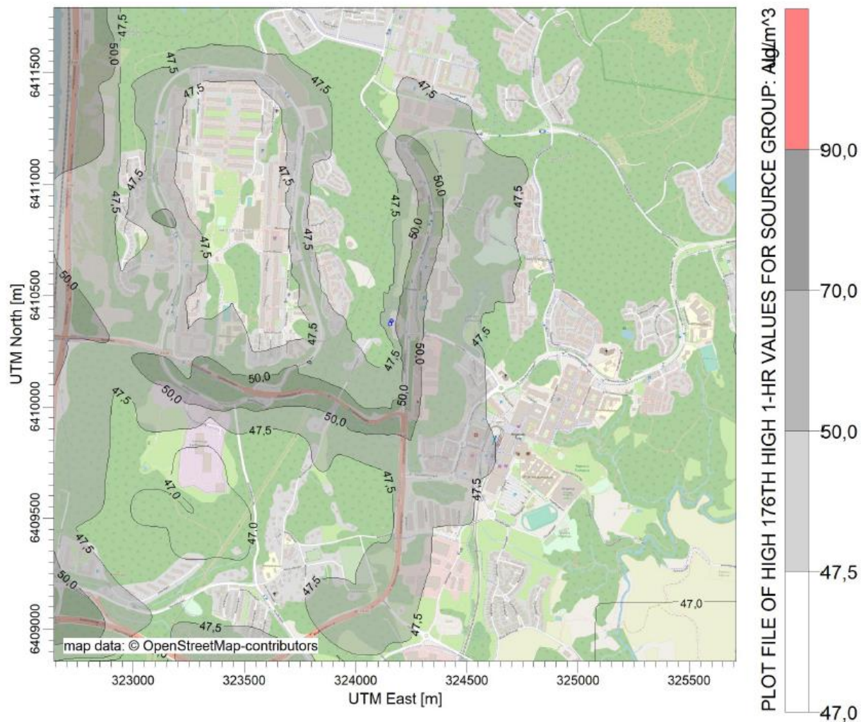
Figur 10: Timmedelvärde (98-percentil) av totalhalt av NO 2 för nollalternativet. Gränsvärdet i MKN överskrids ej.
