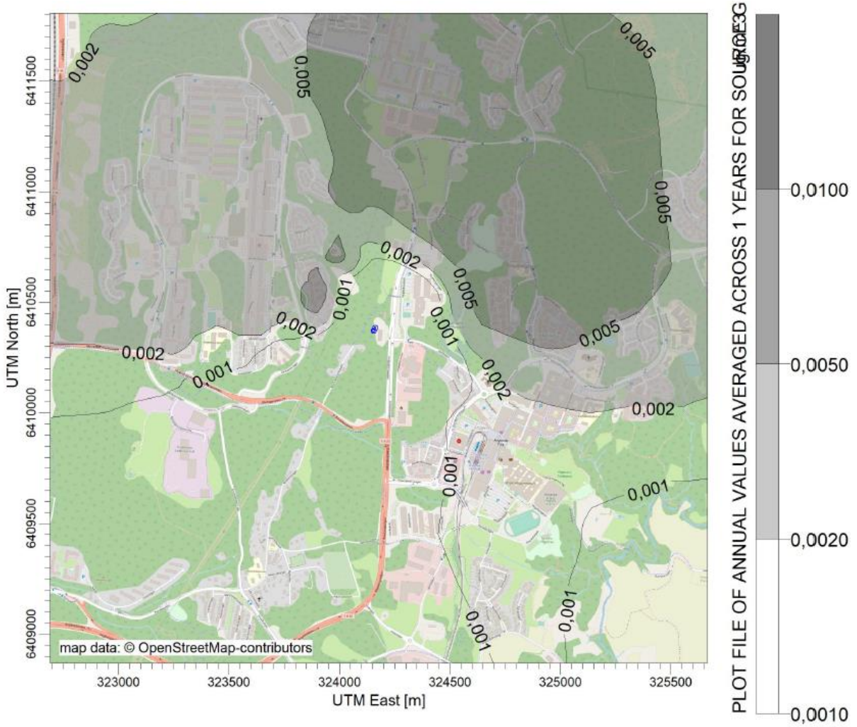
Figur 29: Haltbidrag av PM10 (årsmedel) från existerande anläggning, utan trafik och bakgrundshalter.
