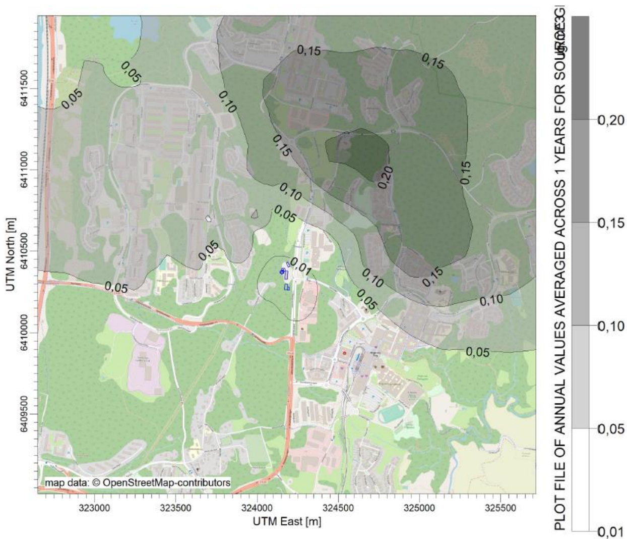
Figur 23: Haltbidrag av NO 2 (årsmedel) från ny anläggning med 100 m skorsten. Haltbidraget inkluderar både existerande skorstenar och ny skorsten.
