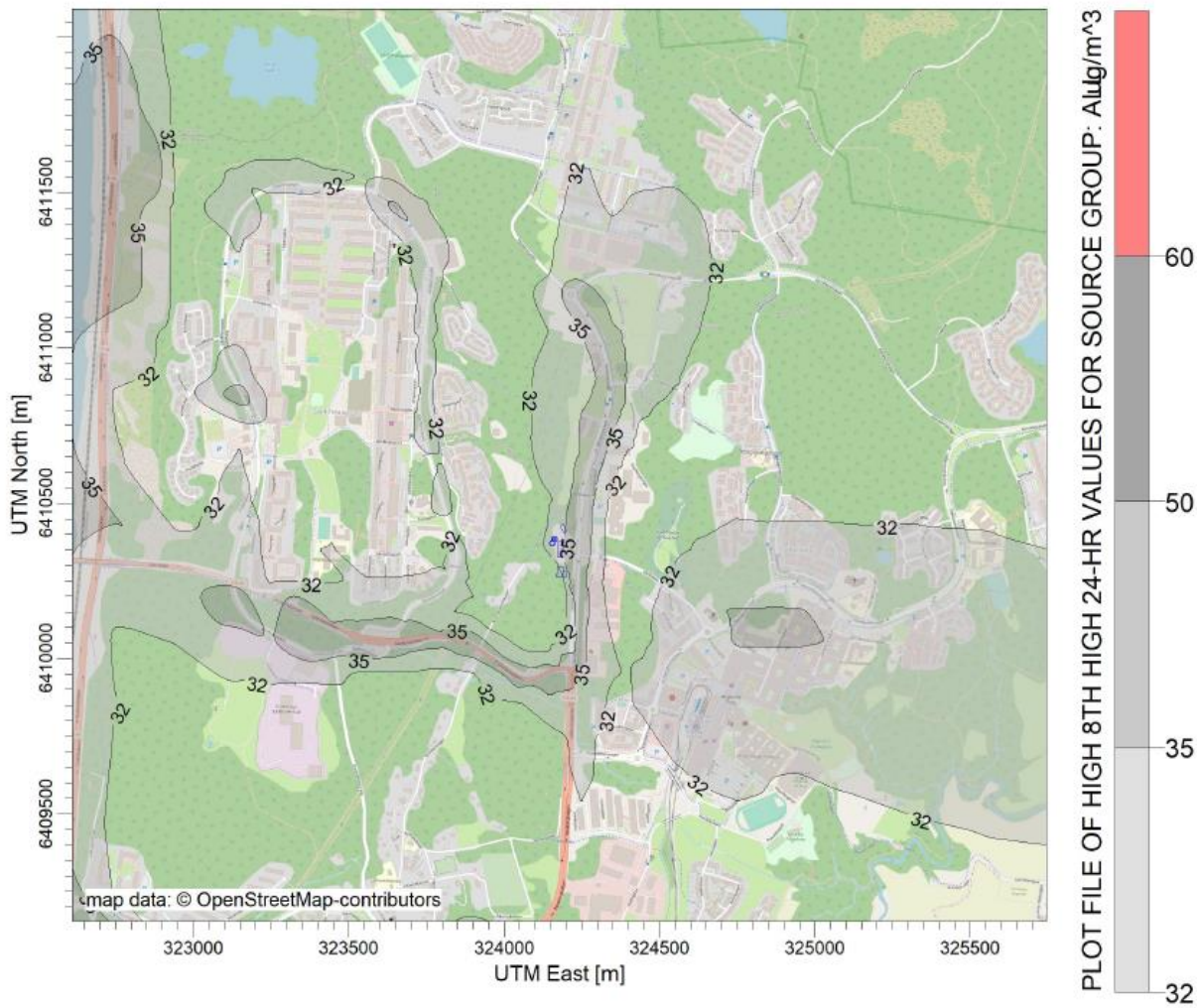
Figur 18: Dygnmedelvärde av totalhalt för NO 2 för utredningsalternativet med 70 m hög skorsten. MKN överskrids ej.
