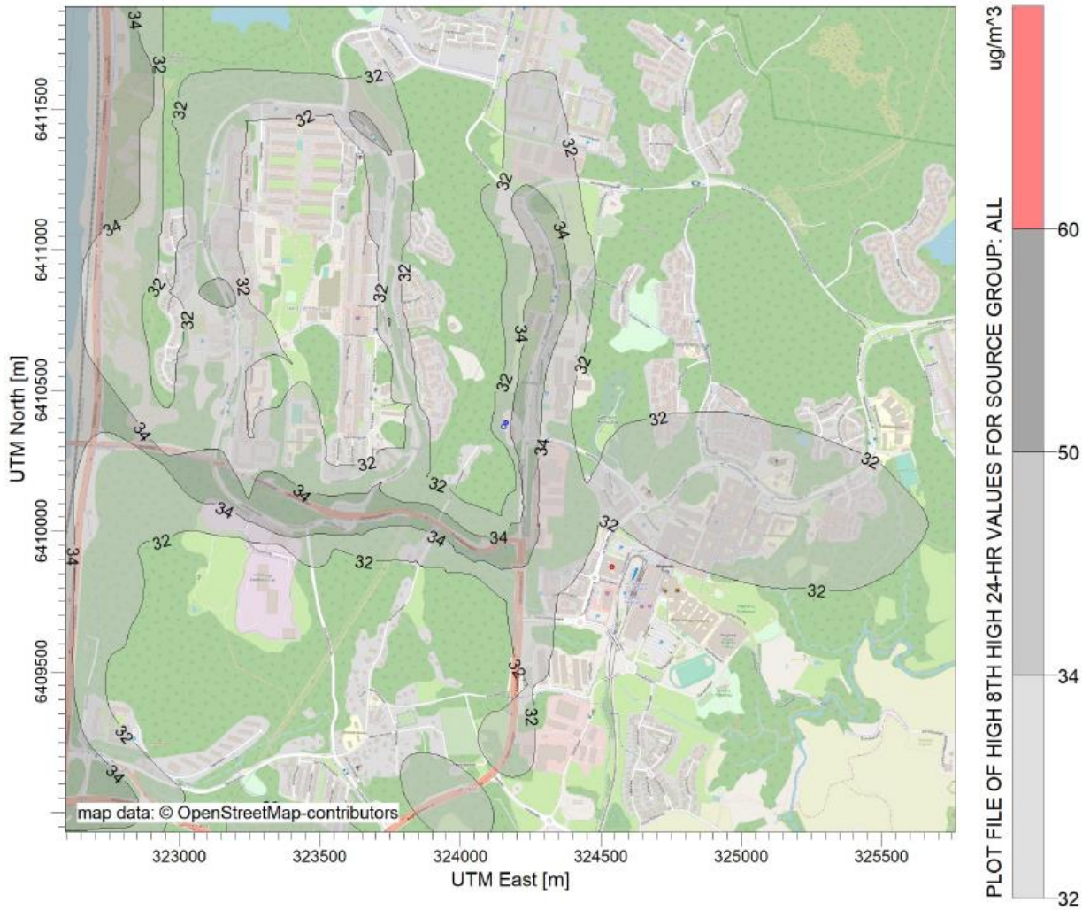
Figur 9: Dygnsmedelvärde (98-percentil) av totalhalt för NO 2 i µg/m 3 för nollalternativet. Gränsvärdet i MKN överskrids ej.
