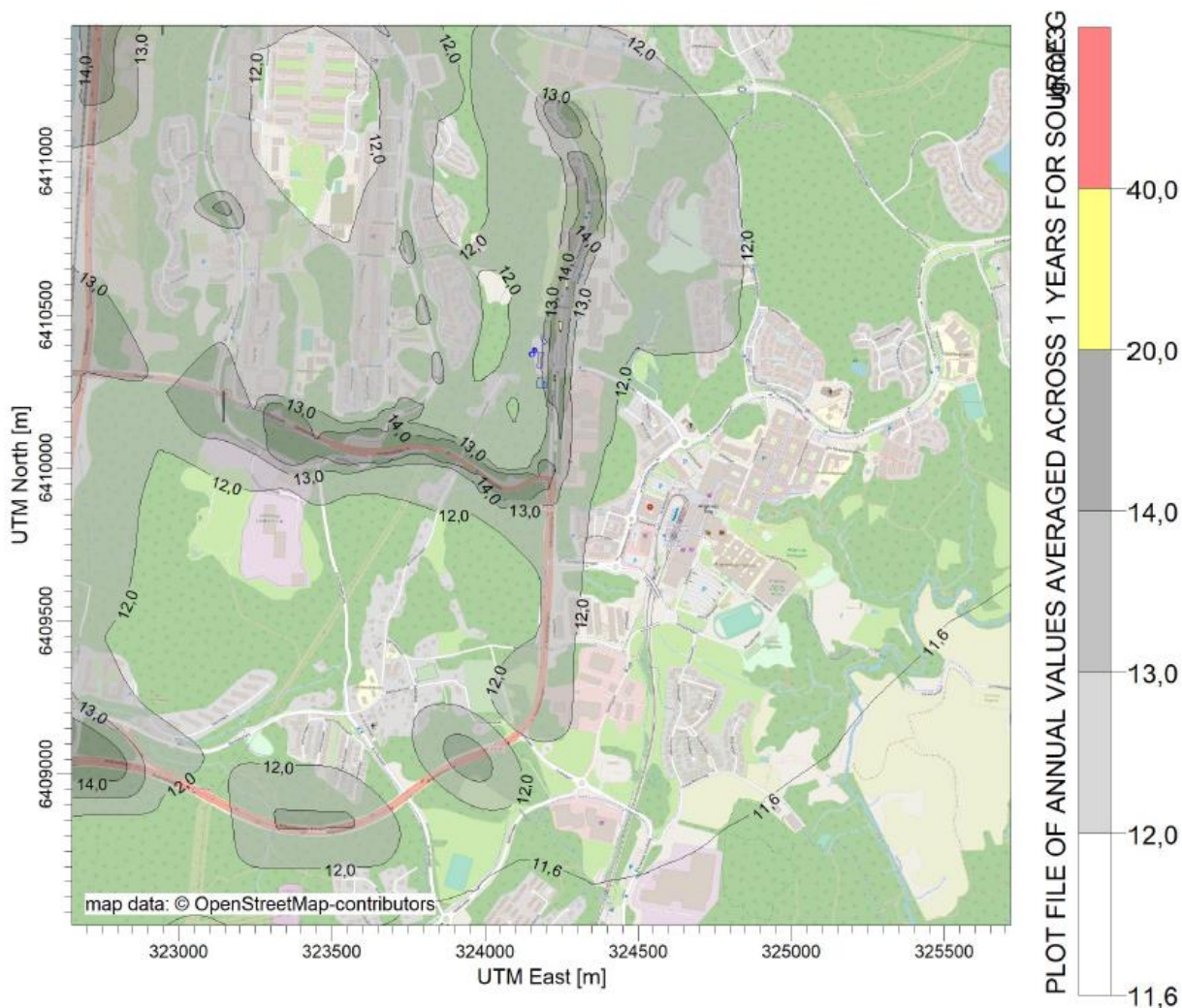
Figur 14: Årsmedelvärde av totalhalt för NO 2 för utredningsalternativet med 70 m hög skorsten. Göteborgs Stads miljömål (gul markering) överskrids i delar av väglinjen nordost om existerande anläggning. MKN överskrids ej.
