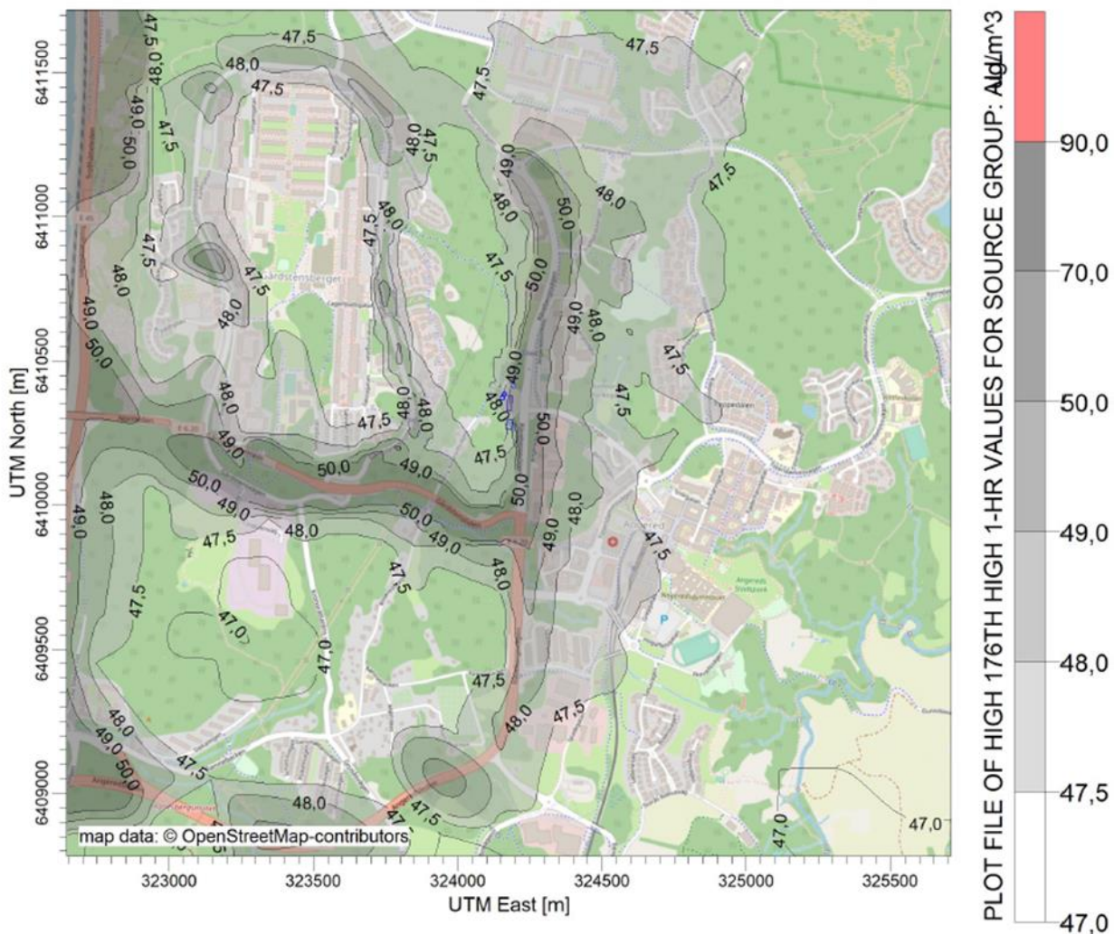
Figur 17: Timmesmedelvärde av totalhalt för NO 2 för utredningsalternativet med 100 m hög skorsten. MKN överskrids ej.
