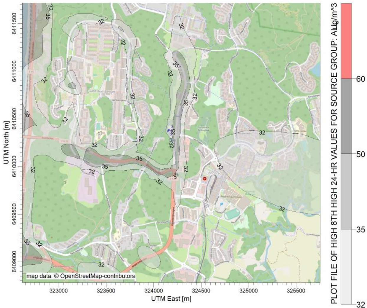
Figur 19: Dygnsmedelvärde av totalhalt för NO 2 för utredningsalternativet med 100 m hög skorsten. MKN överskrids ej.
