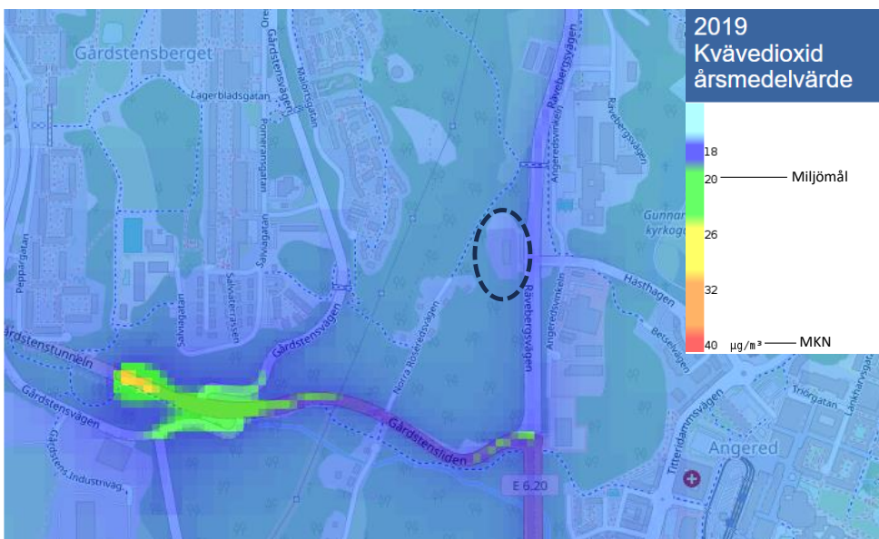
Figur 4. Årsmedelvärde av NO 2 vid värmeverket i Angered (Göteborgs Stad, 2024). Placering av värmeverket vid svart ring.
