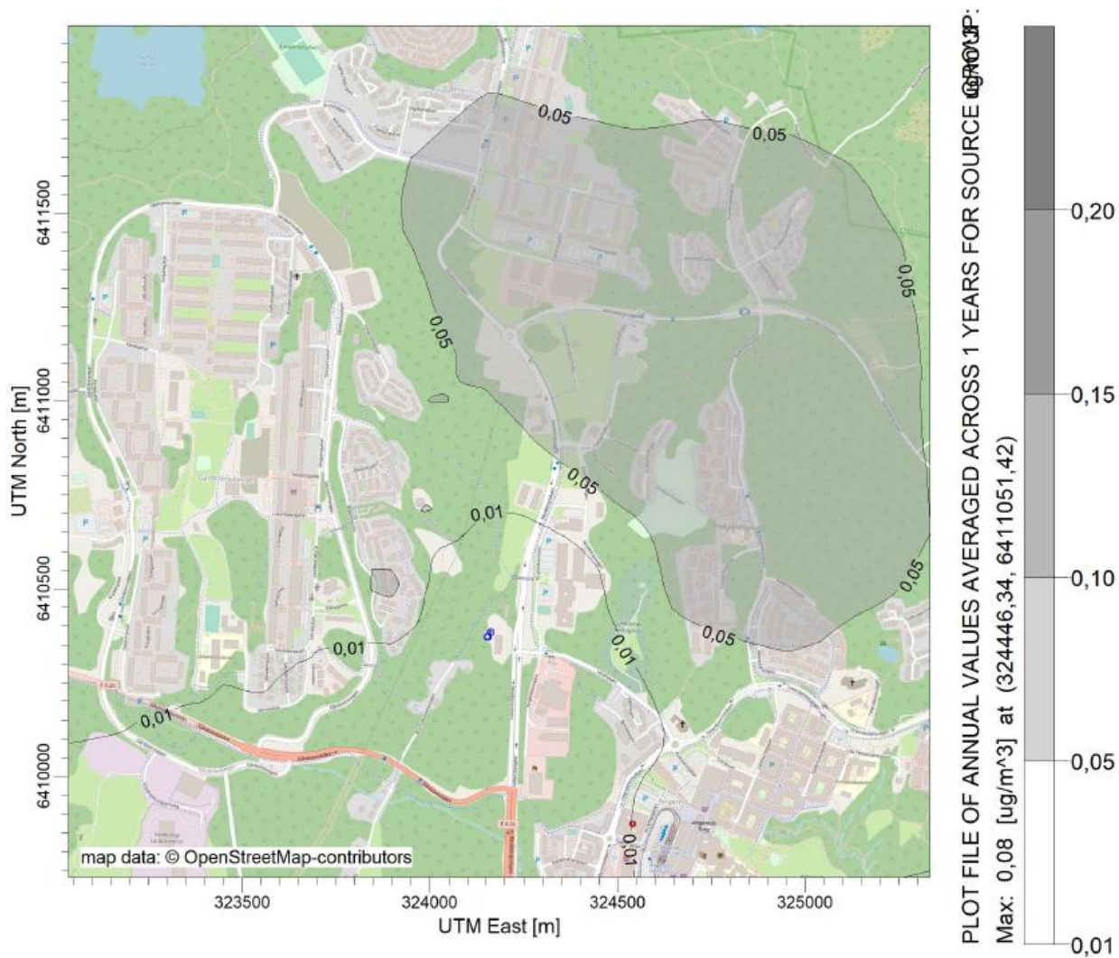
Figur 11: Haltbidrag av NO 2 (årsmedel) från existerande anläggning, utan trafik och bakgrundshalter.
