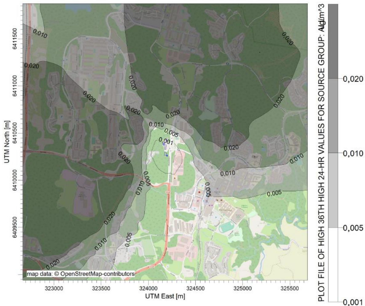
Figur 32: Haltbidrag av partiklar (dygnmedel) från ny anläggning med 70 m skorsten. Haltbidraget inkluderar både existerande skorstenar och ny skorsten, men inte trafik och bakgrundshalter.
