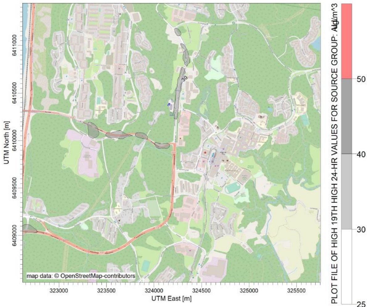
Figur 37: Dygnmedelvärde av totalhalt för NO 2 för planalternativet med 70 m hög skorsten, visat med nya gränsvärden i EU:s reviderade luftkvalitetsdirektiv.
