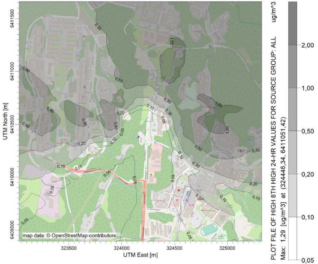
Figur 12: Haltbidrag av NO 2 (dygnmedel) för existerande anläggning, utan trafik och bakgrundshalter.
