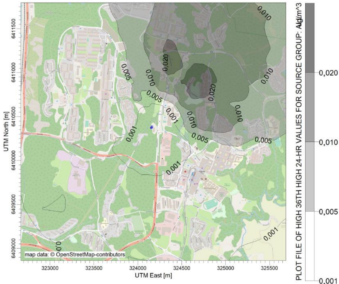
Figur 28: Haltbidrag av PM10 (dygnmedel) från existerande anläggning, utan trafik och bakgrundshalter.
