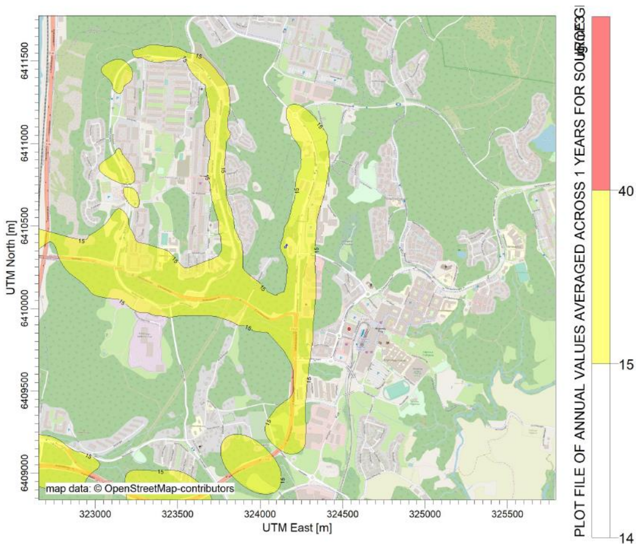
Figur 27: Årsmedelvärde av totalhalt för partiklar för nollalternativet. MKN överskrids ej. Längs vägbanan överskrids Göteborgs stads miljömål för frisk luft.
