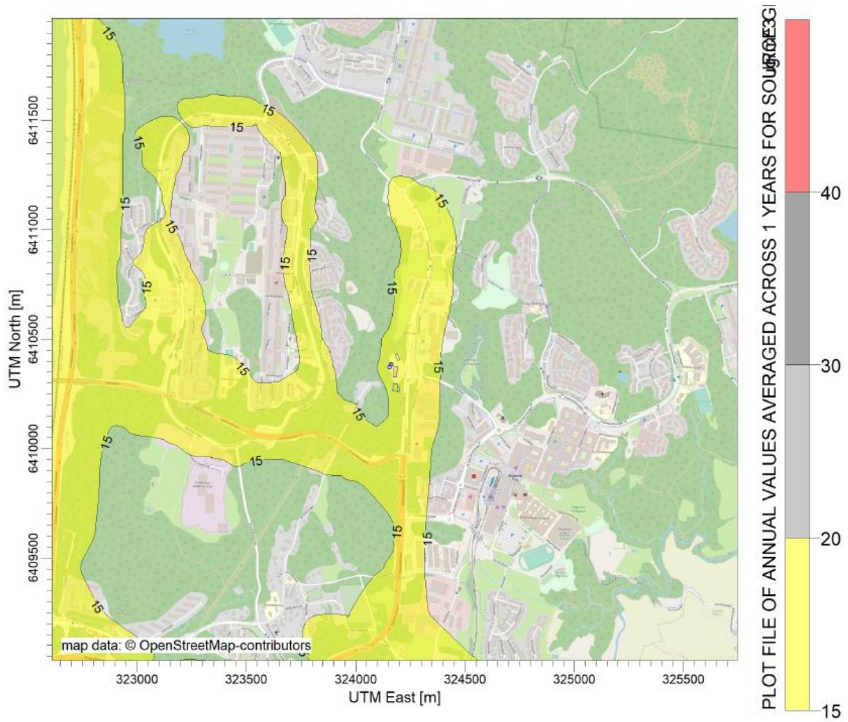
Figur 31: Årsmedelvärde av totalhalt för partiklar för utredningsalternativet vid 70 m hög skorsten. MKN överskrids ej. Längs vägbanan överskrids Göteborgs stads miljömål för utomhusluft.
