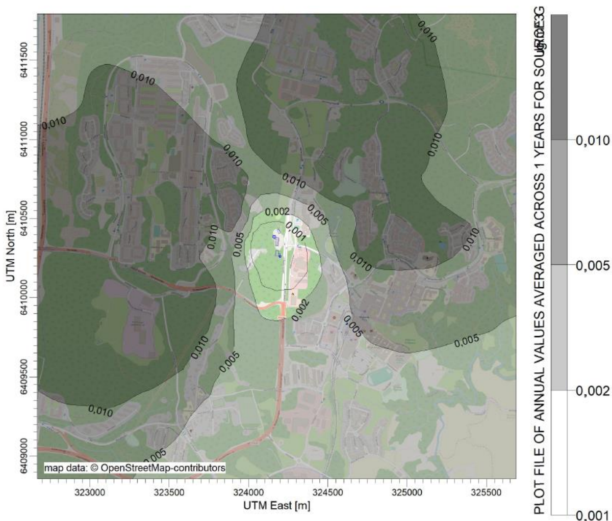
Figur 33: Haltbidrag av partiklar (årsmedel) från ny anläggning med 70 m skorsten. Haltbidraget inkluderar både existerande skorstenar och ny skorsten men inte trafik och bakgrundshalter.
