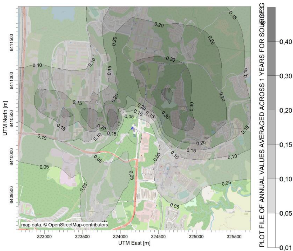
Figur 20: Haltbidrag av NO 2 (årsmedel) från ny anläggning med 70 m skorsten. Haltbidraget inkluderar både existerande skorstenar och ny skorsten men utan trafik och bakgrundshalter.
