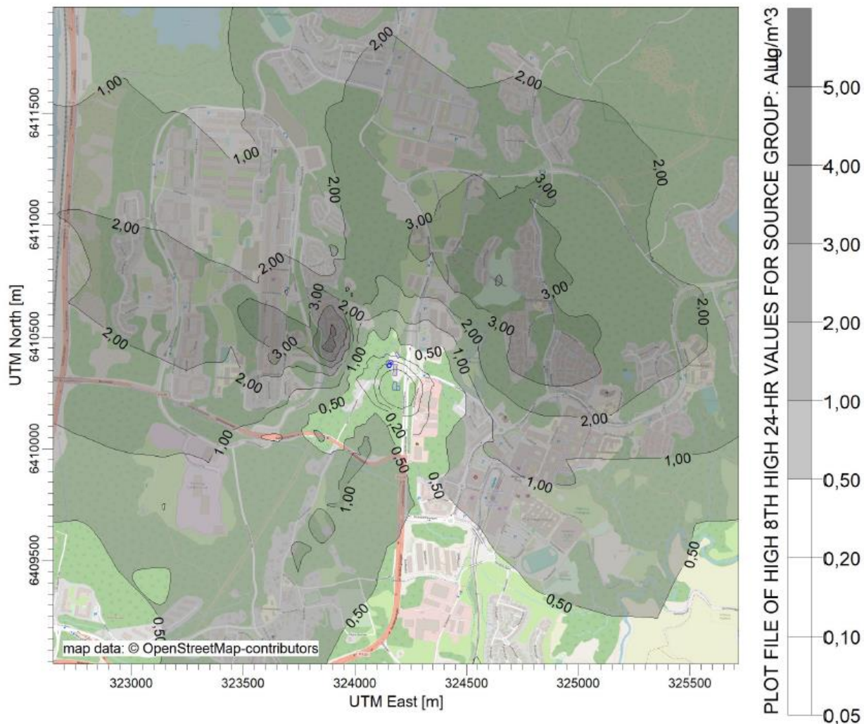
Figur 21: Haltbidrag av NO2 (dygnmedel) från ny anläggning med 70 m skorsten. Haltbidraget inkluderar både existerande skorstenar och ny skorsten men är utan trafik och bakgrundshalter.
