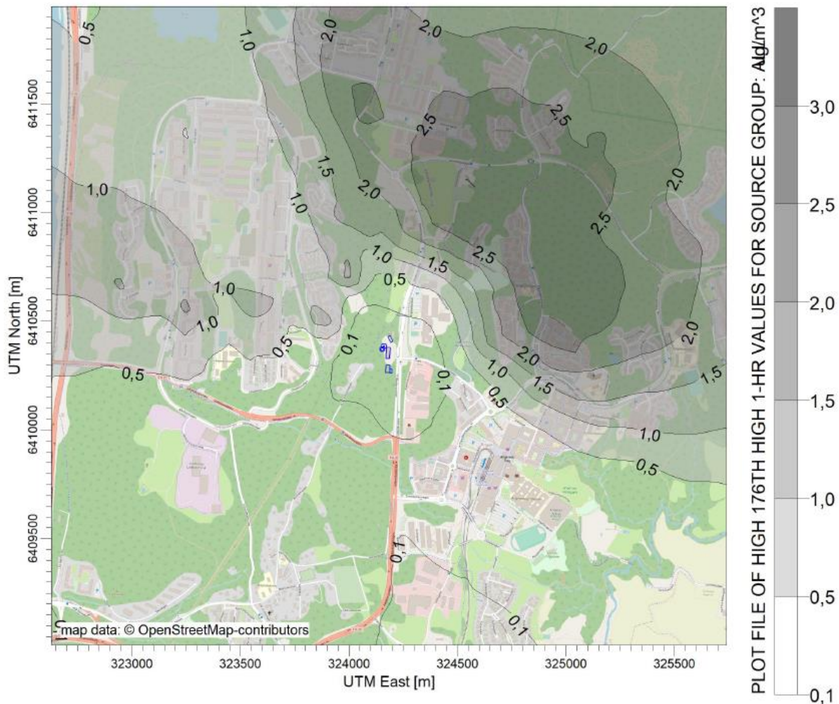
Figur 25: Haltbidrag av NO2 (timmesmedel) från ny anläggning med 100 m skorsten. Haltbidraget inkluderar både existerande skorstenar och ny skorsten.
