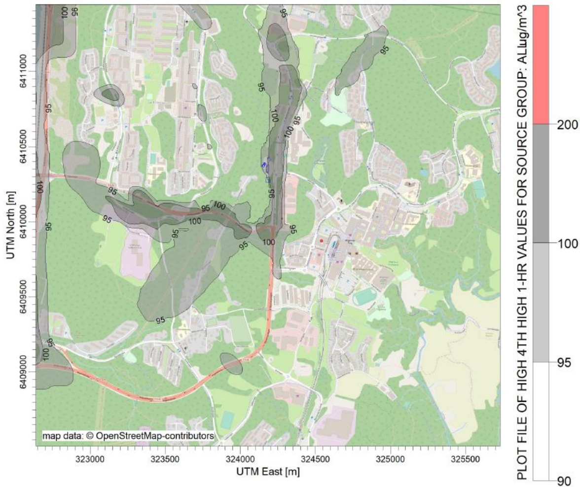
Figur 36: Timmesmedelvärde av totalhalt för NO 2 för planalternativet med 70 m hög skorsten, visat med nya gränsvärden i EU:s reviderade luftkvalitetsdirektiv.
