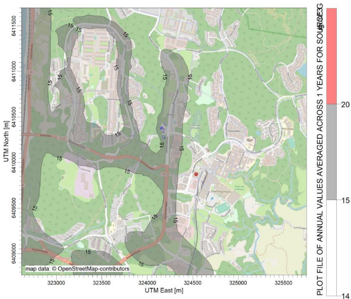
Figur 35: Årsmedelvärde av totalhalt för partiklar för planalternativet med 70 m hög skorsten, visat med nya gränsvärden i EU:s reviderade luftkvalitetsdirektiv.
